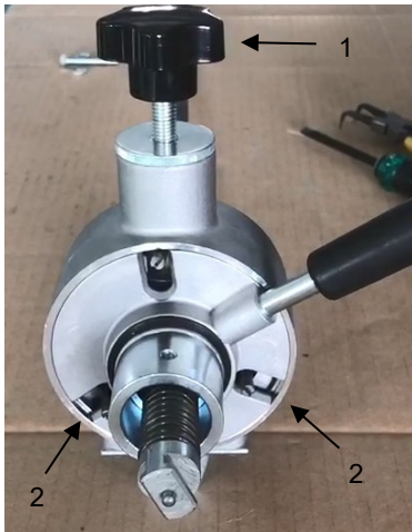
Fig. 35: unité d'avance, palier marqué d'une flèche
